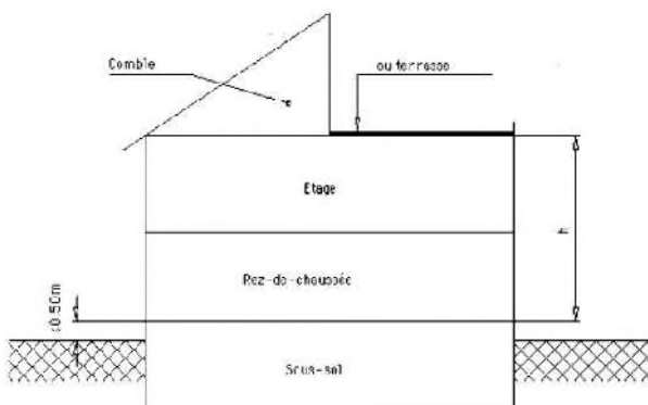
Coupe sur bâtiment (terrain plat)
