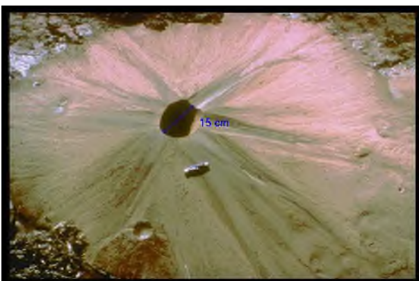
Volcans de boue ©USGS, BRGM
