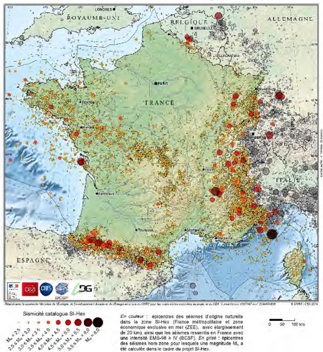
Carte de sismicité de la France ©BCSF
