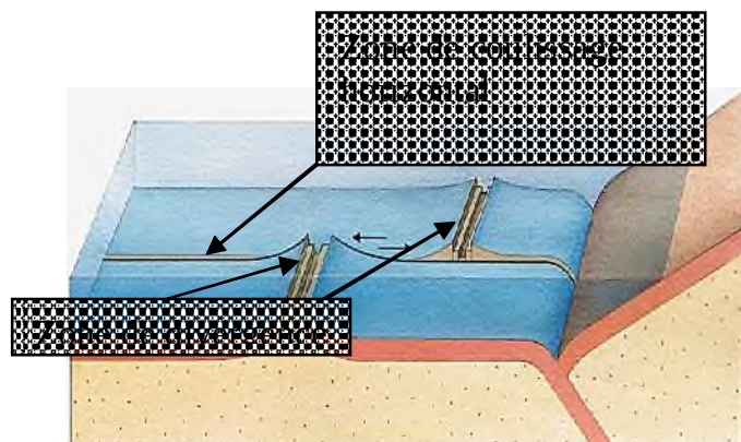
Faille transformante – Dorsale océanique ©Larousse
