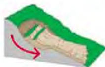
Glissement de terrain
