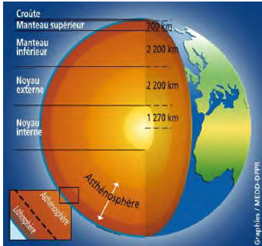
Structure interne de la Terre
