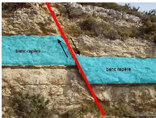
Rejet - Faille normale
