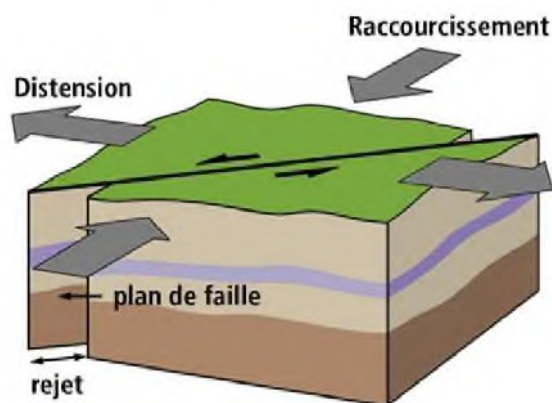
Faille décrochante © BRGM
